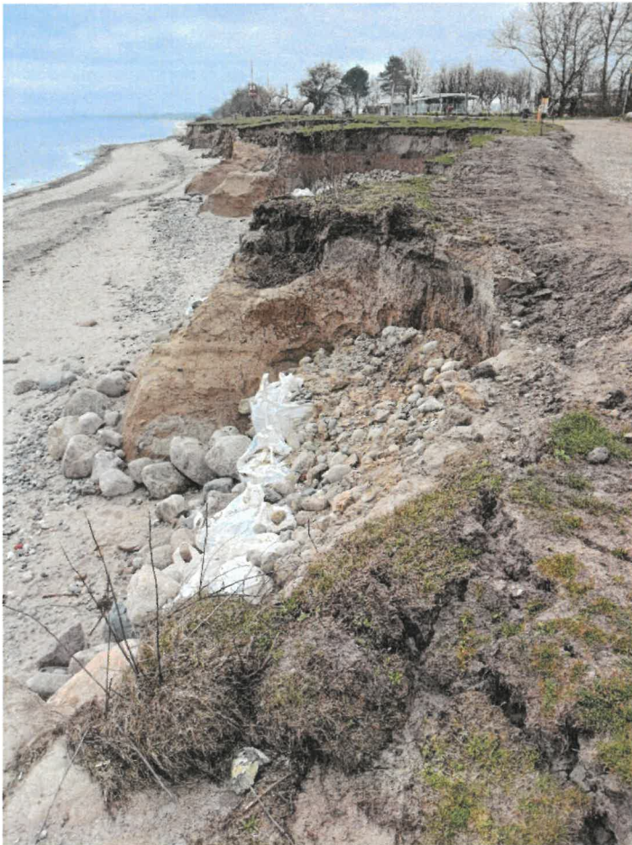
Schäden im Baubereich Süd nach der Sturmflut im Oktober 2023.
