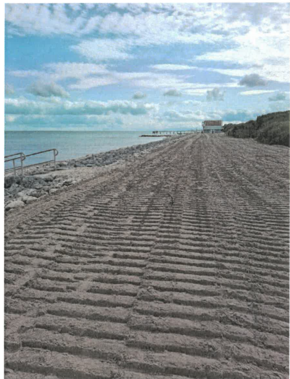
Wiederherstellung Bereich der „Graudüne“ – letzte Arbeitsgänge im Baubereich Nord im September 2025
